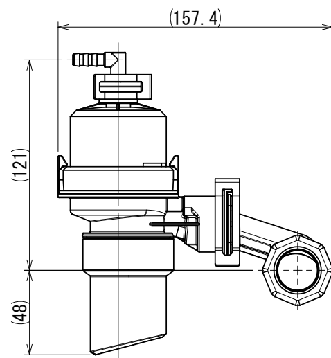
差し込みソケット水平取付図 注4
