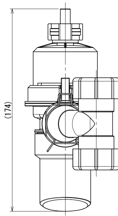
右側面図
