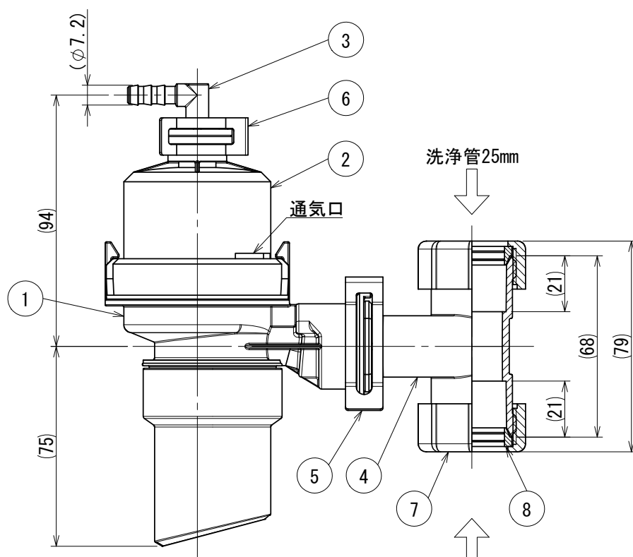
正面図
