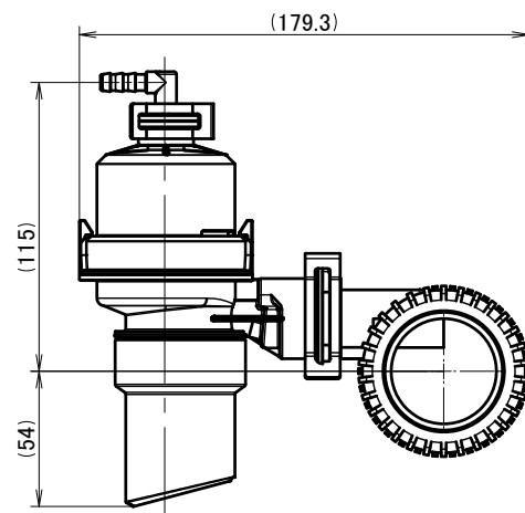
差し込みソケット水平取付図 注4
