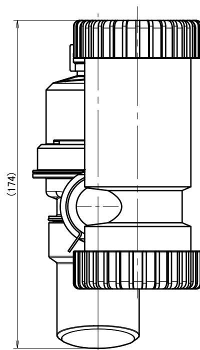
右側面図
