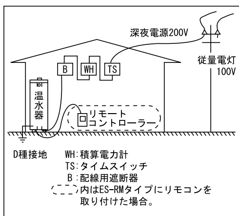
図1 深夜電力の場合
