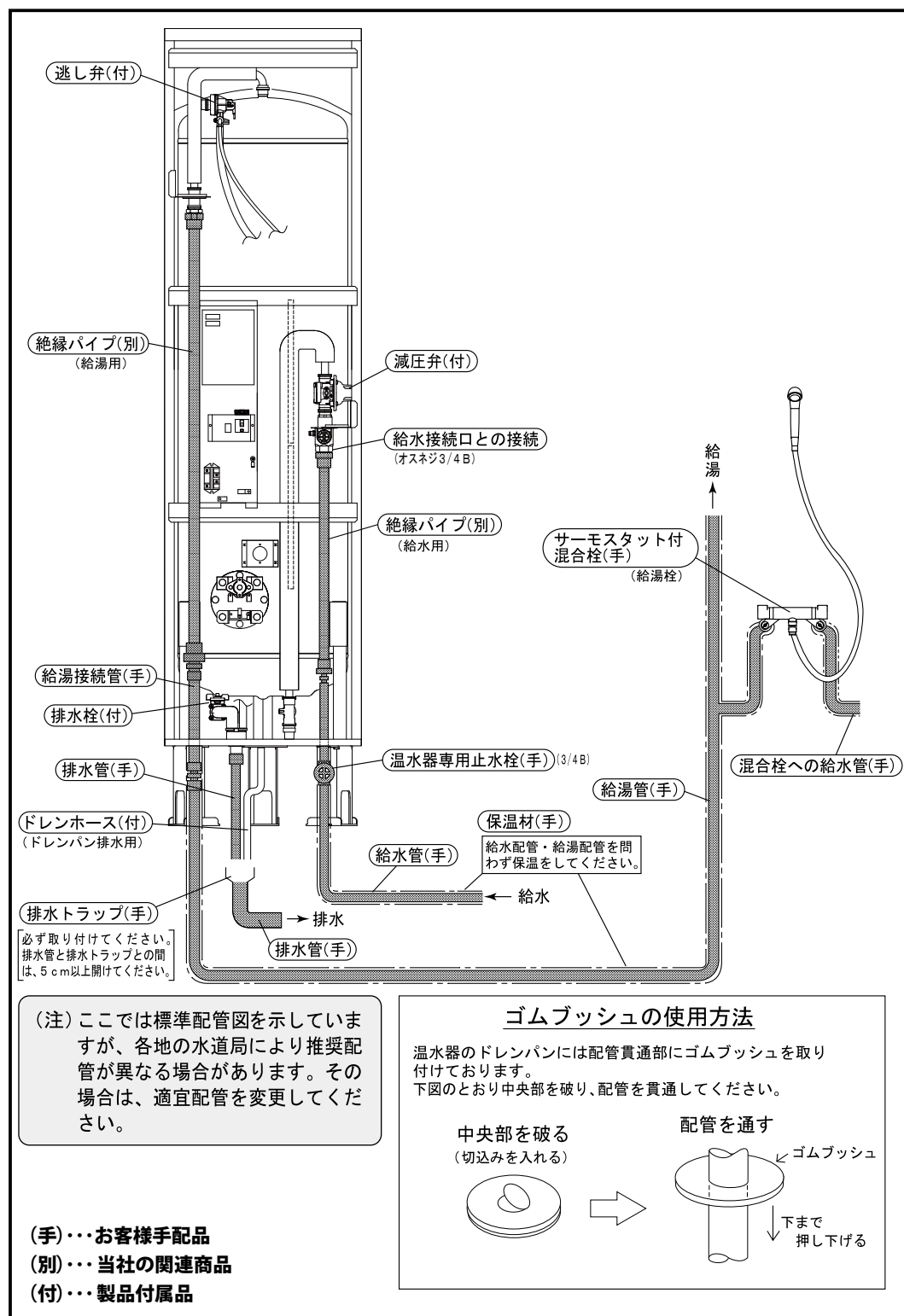
標準配管図 (図はES-150RM)
