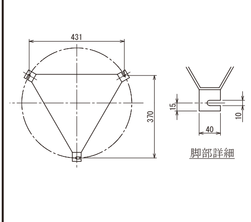
【本体固定寸法図】
