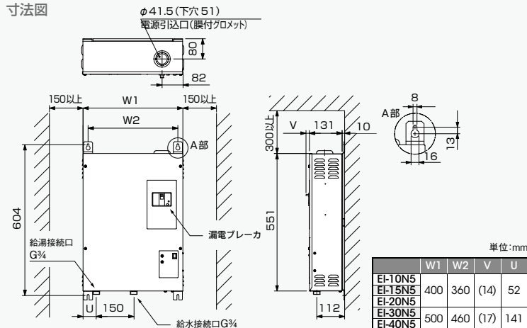
寸法図
