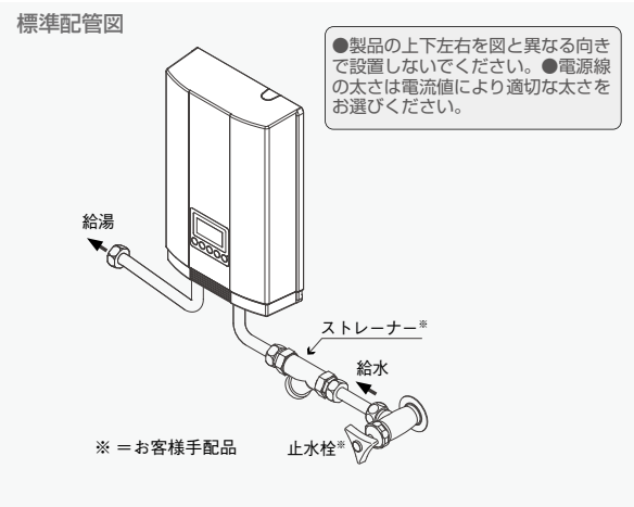
標準配管図
