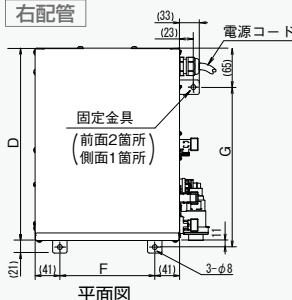
右配管
