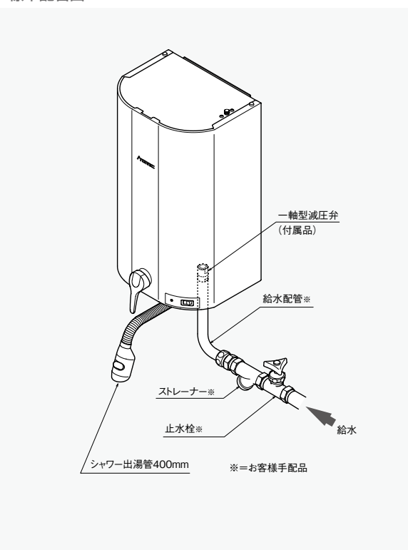
標準配管図
