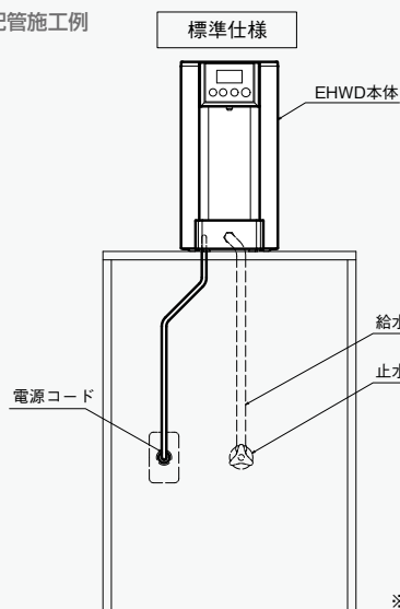
配管施工例
