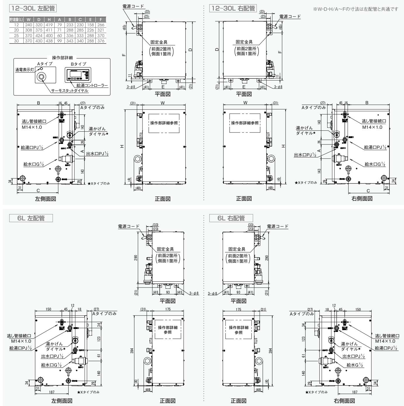
寸法図 ESN
