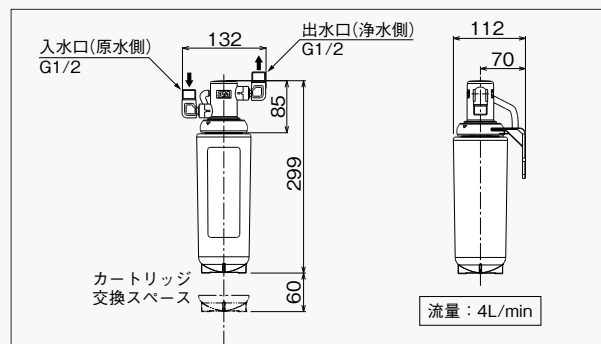
净水器寸法図
