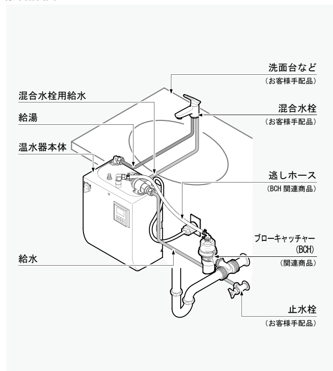
標準配管図
