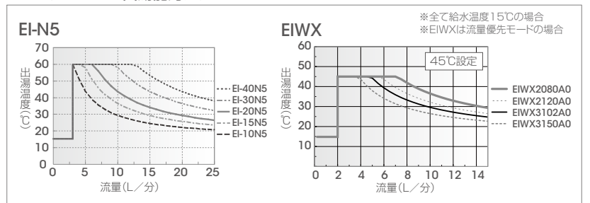
EI-N5 / EIWX 出湯能力グラフ
