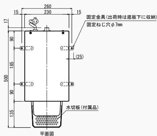
寸法図 EHWD-14
