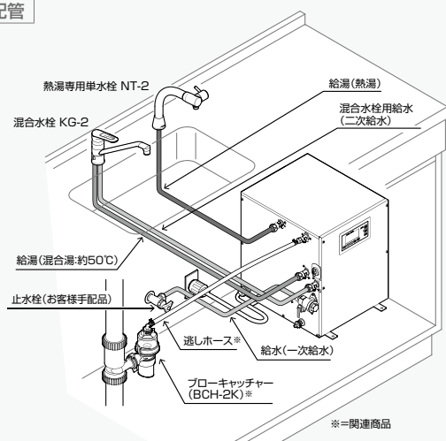
左配管
