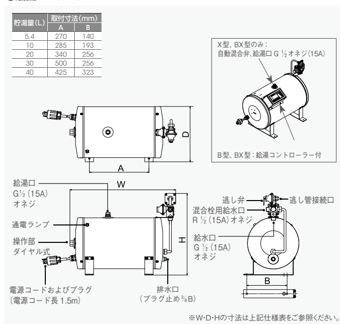
寸法図 ES-N3
