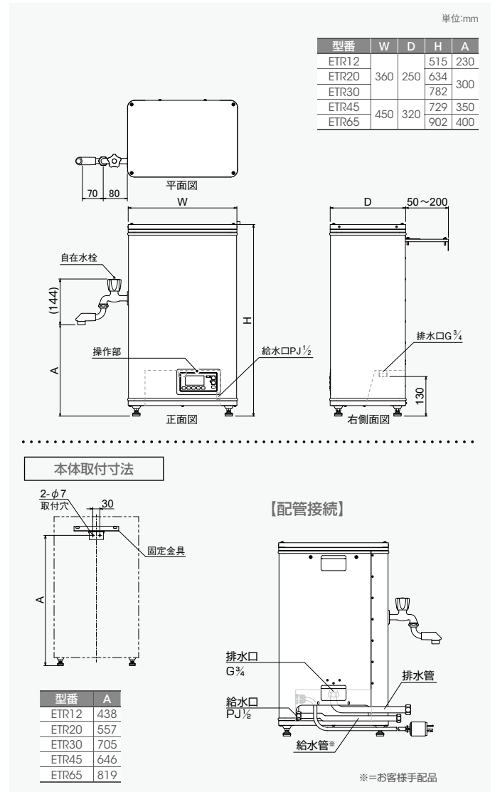
寸法図 ETR
