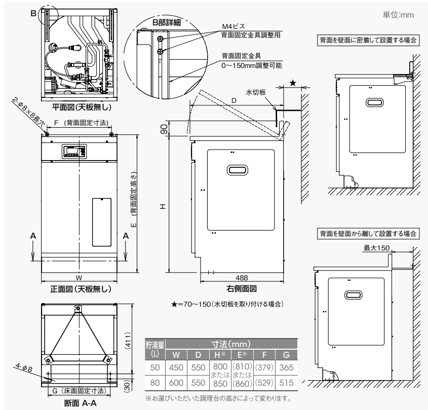
寸法図 ES-DWUB
