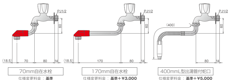
蛇口正面
