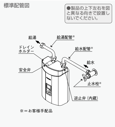
標準配管図
