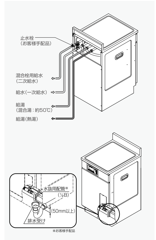
標準配管図
