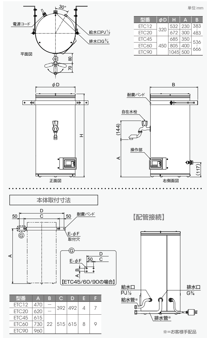
寸法図 ETC
