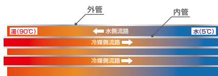
多重管式ガスクラ断面図
