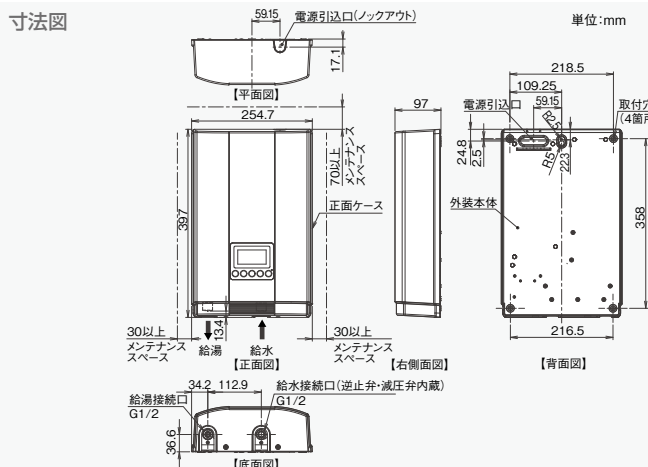
寸法図
