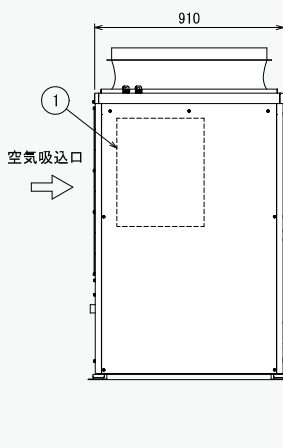
右側面図
