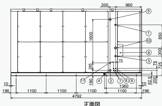
正面図
