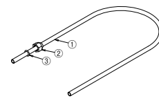
①逃し銅管(L=700mm)×1 ②袋ナットM14×1 ③Oリング×1
