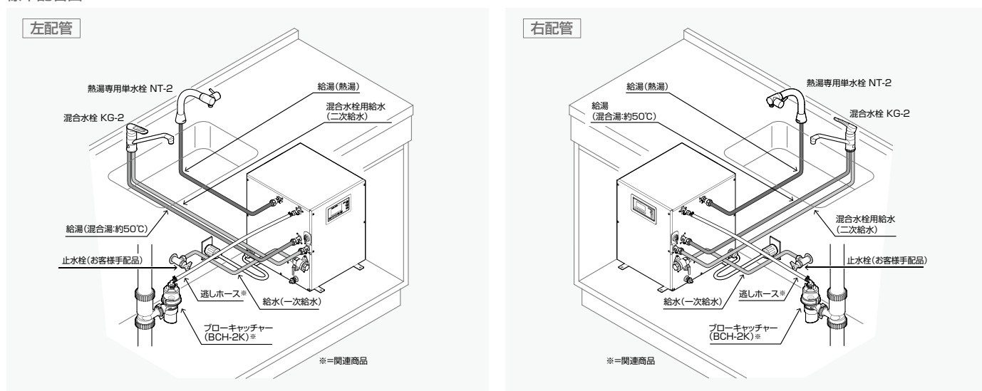
標準配管図 熱湯栓付混合栓MZ-N3Pシリーズと組み合わせる場合はP.117
