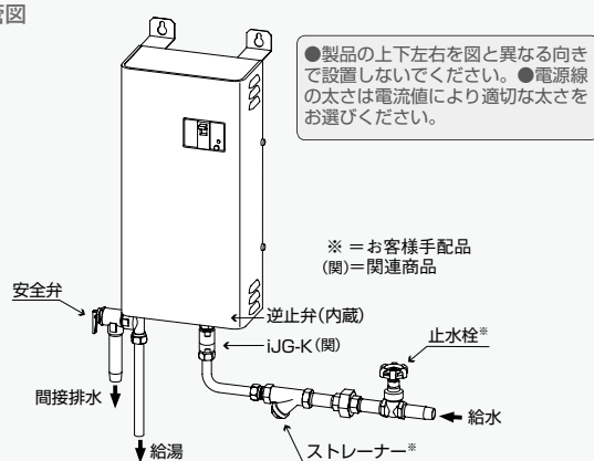
標準配管図
