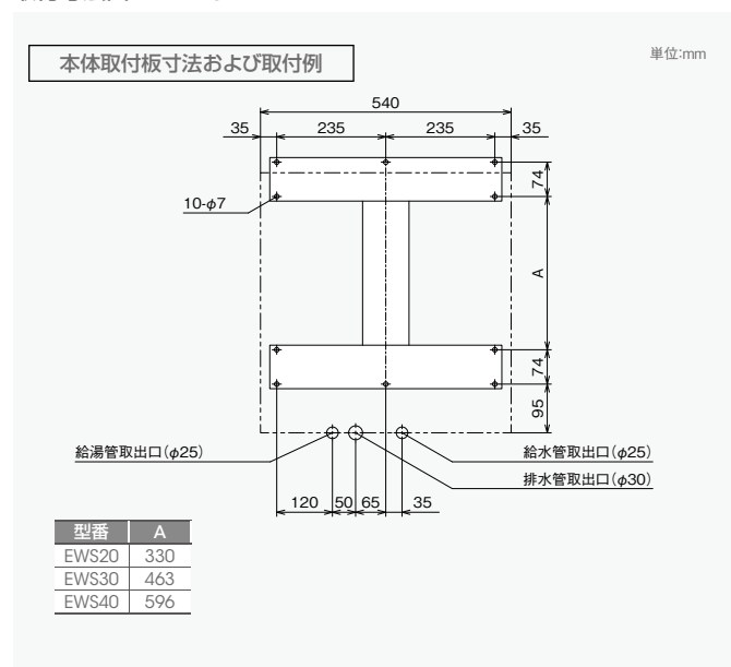
取付寸法図 EWSシリーズ
