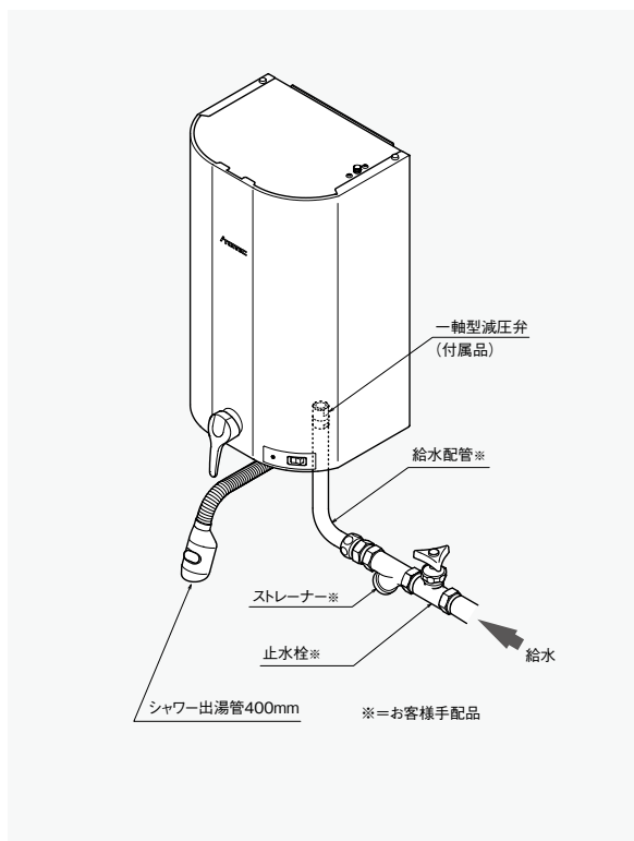
標準配管図
