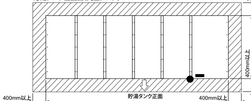
貯湯タンク上面図(高圧タンク)
