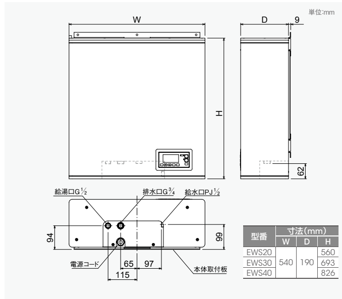
寸法図 EWSシリーズ
