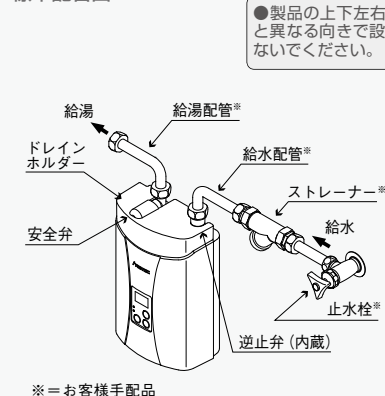
標準配管図
