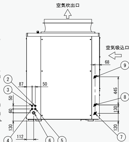
裏面図
