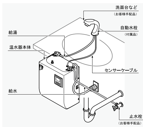
標準配管図
