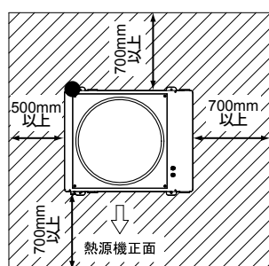
熱源機上面図
