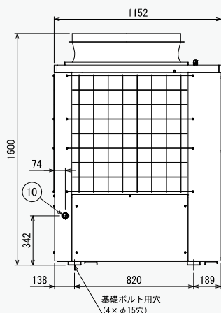
正面図
