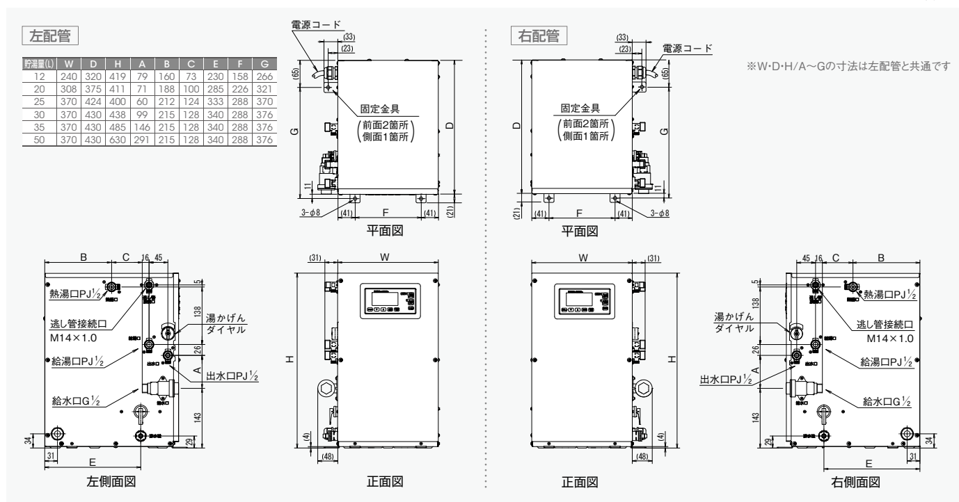
寸法図 ESD
