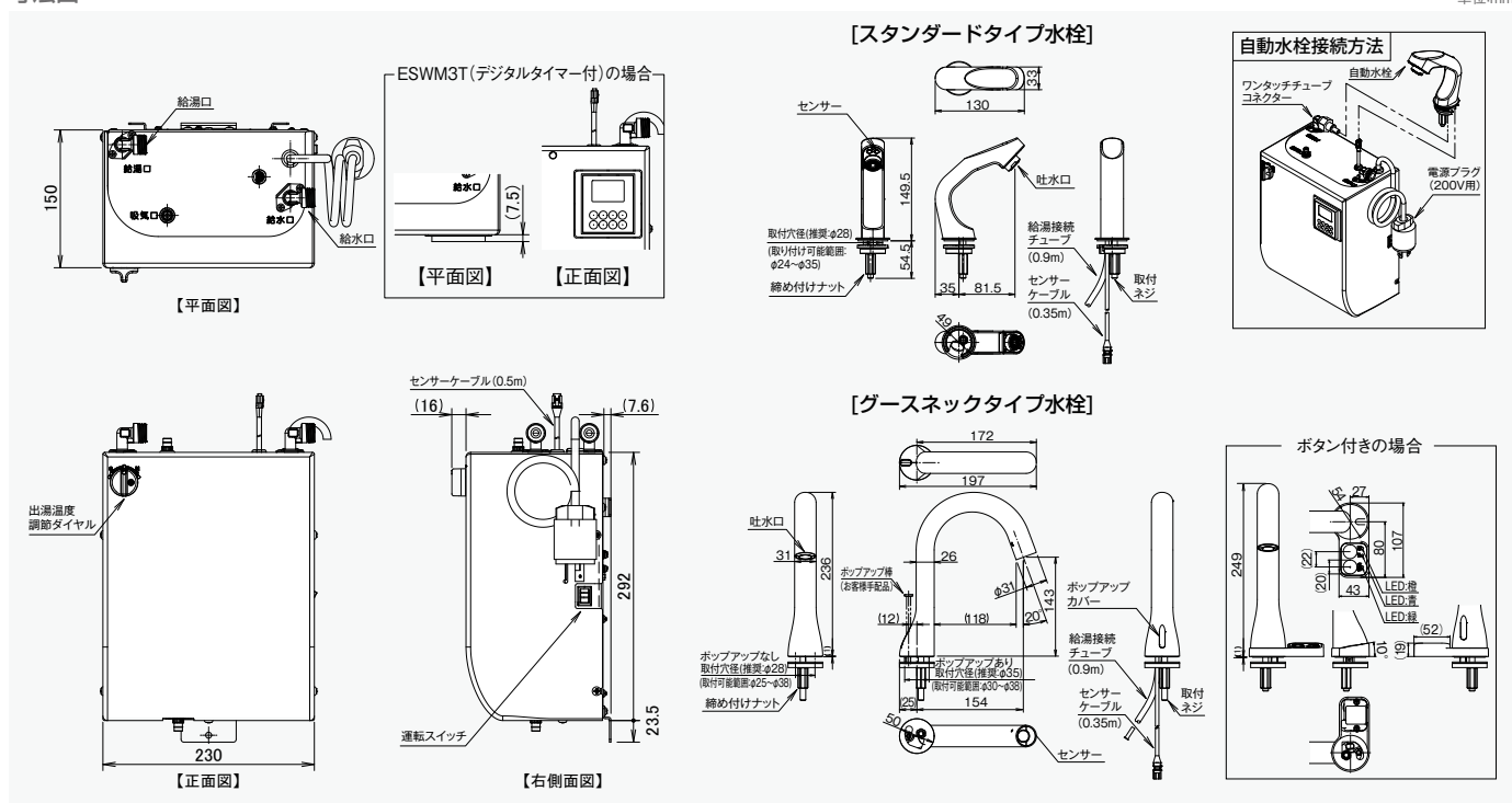
寸法図
