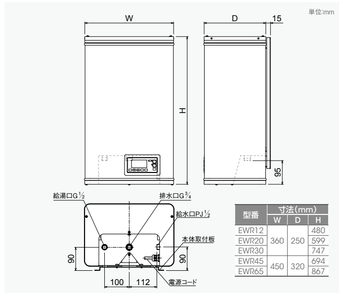
寸法図 EWRシリーズ
