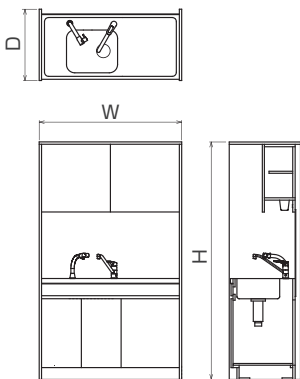
寸法図
