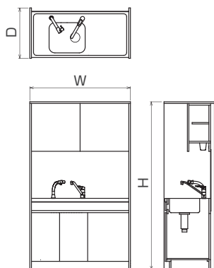
寸法図
