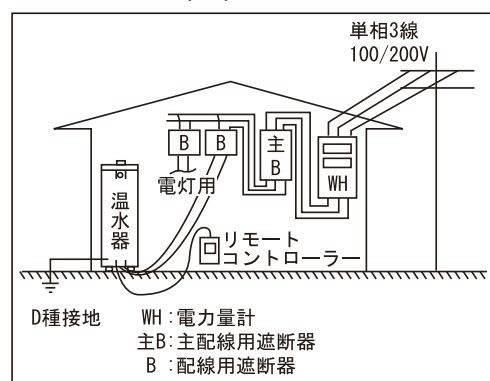
図2 時間帯別電灯/ 季節別時間帯別電灯の場合 ES-RMタイプ+リモコン ES-RMKタイプ
