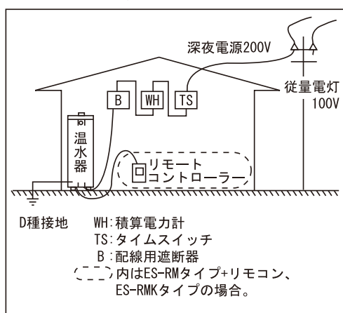
図1 深夜電力の場合 ES-RMタイプ ES-RMタイプ+リモコン ES-RMKタイプ
